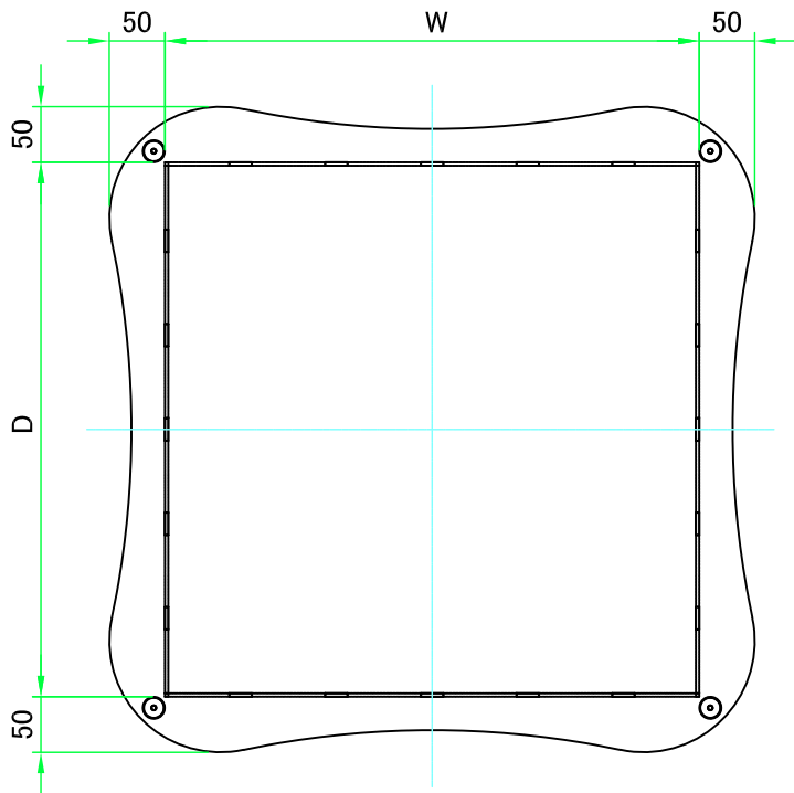
Wパネル1 / W panel 1
