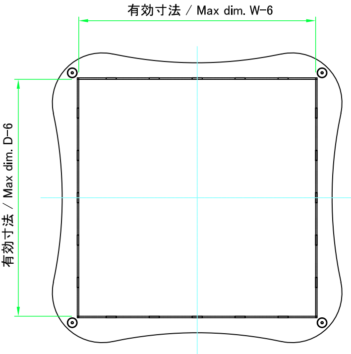
下カバー / Bottom cover
